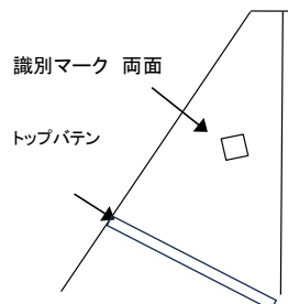
420 級 識別マーク表示位置
