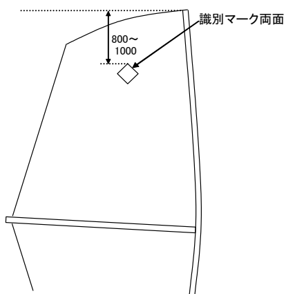
ILCA6級 識別マーク表示位置
