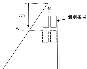
スナイプ級 識別番号表示位置
